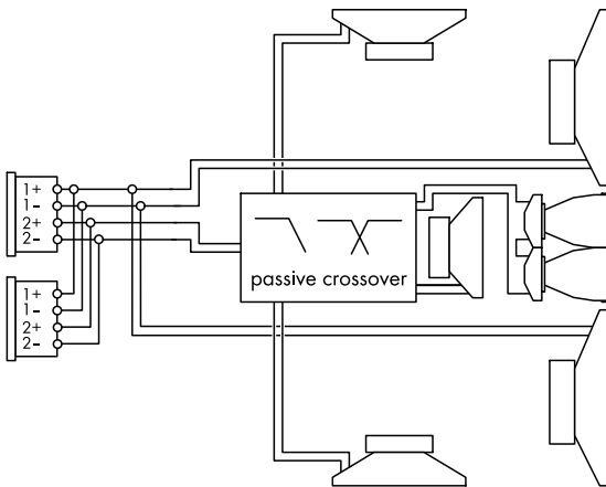
NLT4 F/M Connector wiring
